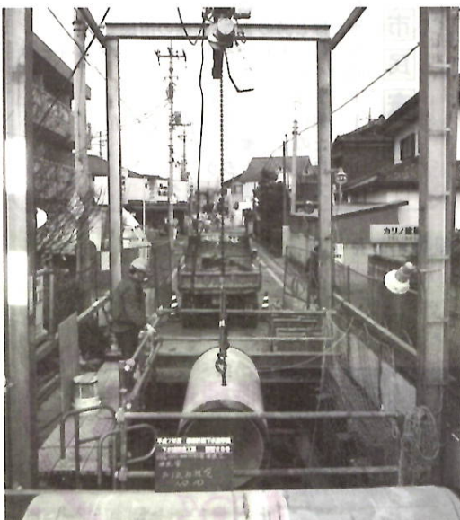
公共下水道を普及させるために着々と進む工事
