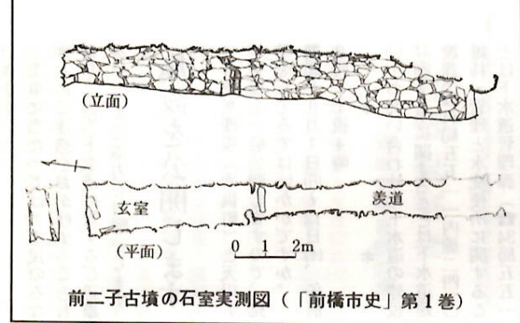
前二子古墳の石室実測図(「前橋市史」第1巻)
