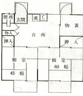
第1種 簡耐平屋建(MTC-C) 36.52㎡
