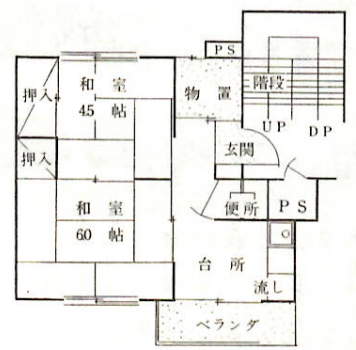
第2種 中耐4階建 41.06㎡
